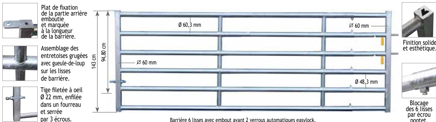
Barrière 6 lisses avec embout avant 2 verrous automatiques easylock.
